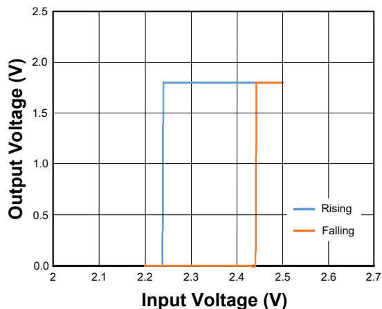
V_{IN} UVLO
